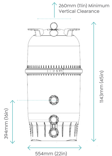
Di 80 Ultra Fine Filter
